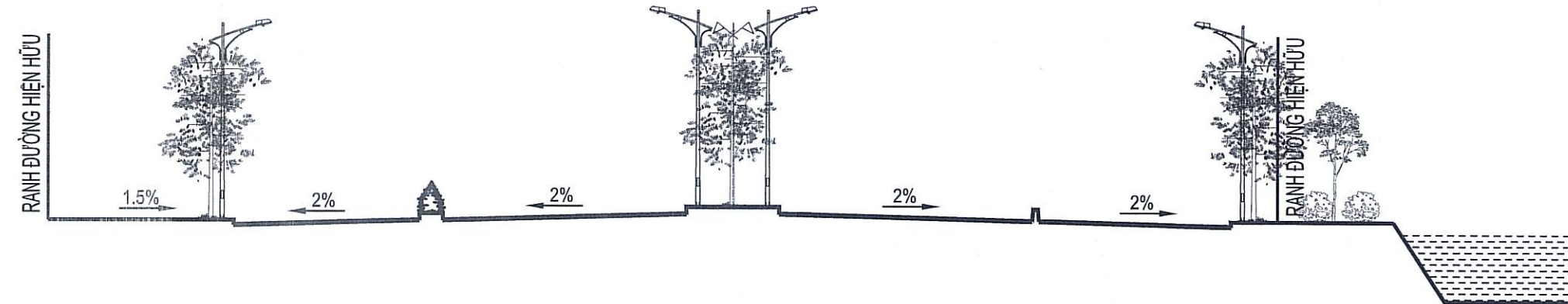
MẶT CẮT 1 - 1 TỶ LỆ 1/250 (ĐƯỜNG VÕ VĂN KIỆT)
