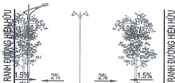
MẶT CẮT 3 - 3 TỶ LỆ 1/250 (ĐƯỜNG YERSIN)
