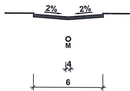
MẶT CẮT 2 - 2
