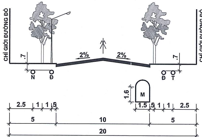
MẶT CẮT 1 - 1
