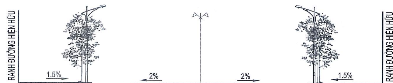
MẶT CẮT 2 - 2 TỶ LỆ 1/250 (ĐƯỜNG NGUYỄN THÁI HỌC)
