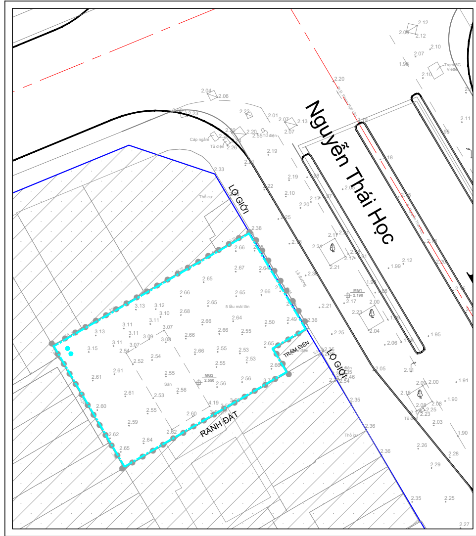
SƠ ĐỒ RANH GIỚI TẦNG HẦM - TỶ LỆ: 1/500
