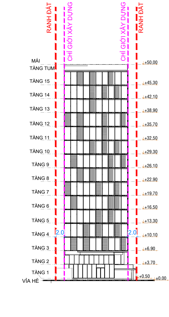
MẶT ĐỨNG - HƯỚNG ĐÔNG BẮC TỶ LỆ 1/500
