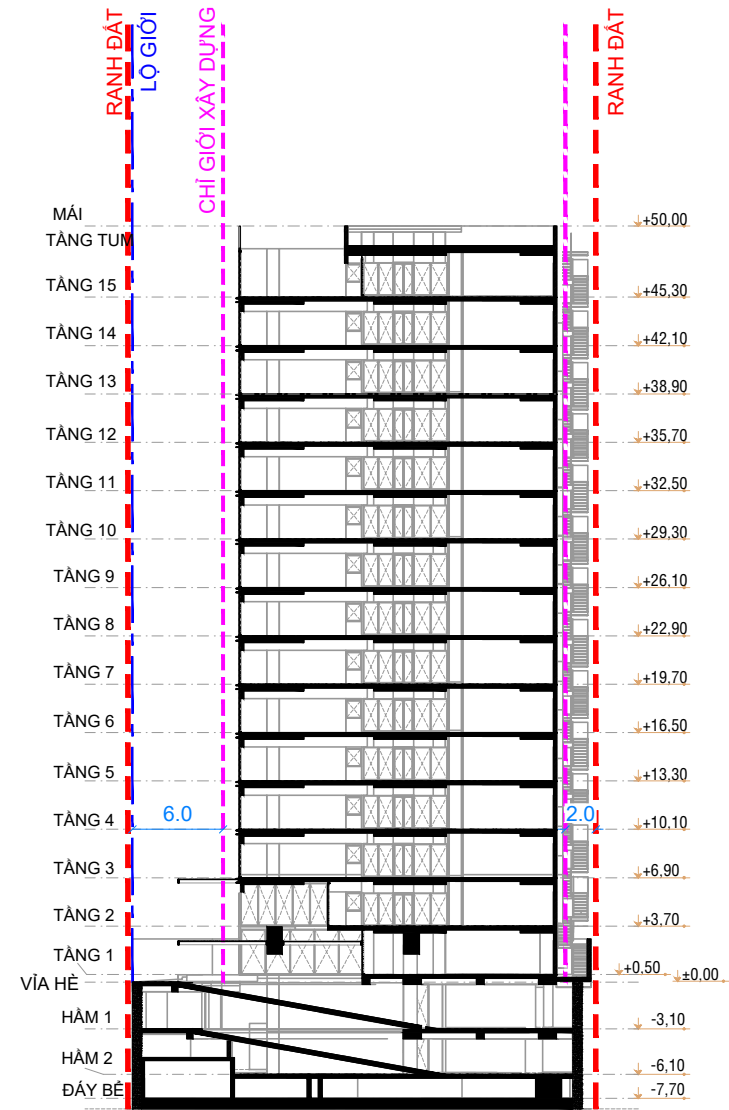
MẶT CẮT MINH HỌA - TỶ LỆ 1/500
